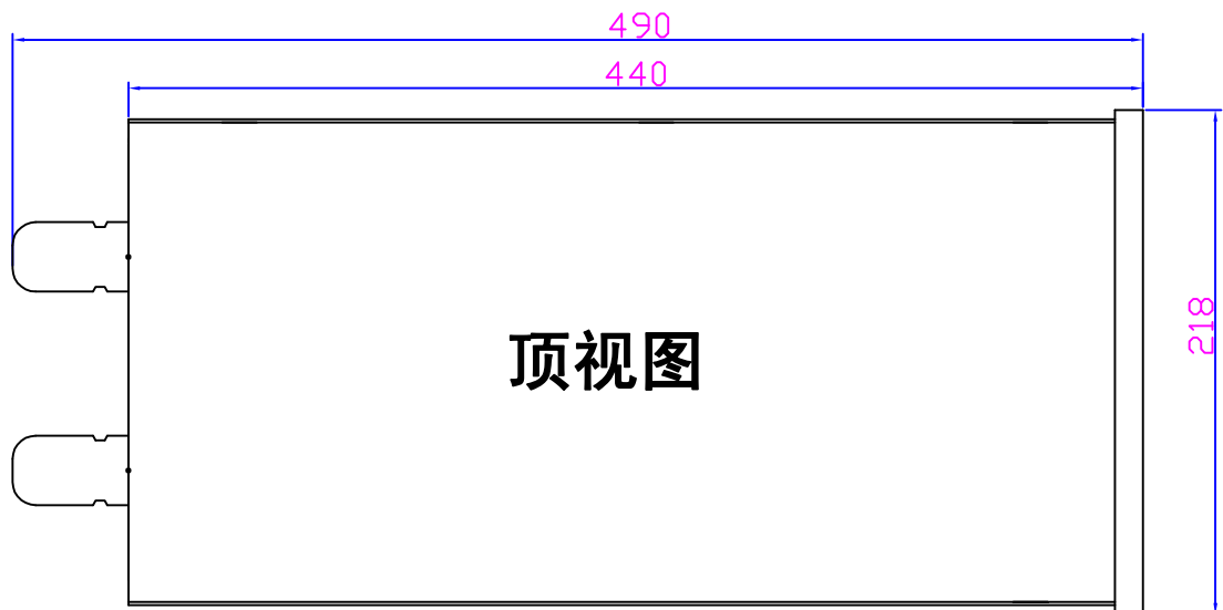
立式4-6K 机箱固定尺寸
